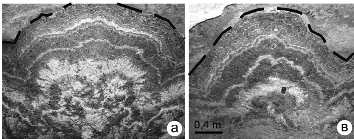
Рис. 2. Куполовидная слоистость средней пачки гипсовой толщи в вертикальном сечении: а) пещера Оптимистическая (фото И.И.Турчинова); б) пещера Мушкарова яма (фото авторов). Пунктирной линией показана верхняя граница средней пачки гипсов, совпадающая с бентонитовым прослоем.
