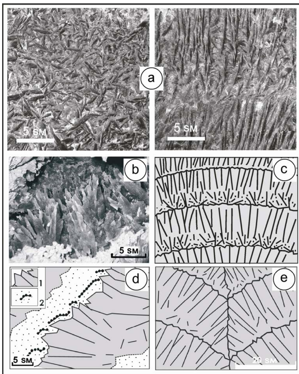
Рис. 3. Структуры и текстуры первичной кристаллизации и осаждения гипсов: a – ориентировка кристаллоагрегатов крупнокристаллического гипса в сечении, параллельном напластованию (левый снимок), в сечении, перпендикулярном напластованию (правый снимок); b – друзовая структура первичного (осадочно-кристаллизационного) медового гипса; c – зональное строение слоев крупно-гигантокристаллического гипса (зоны зачаточного, друзового, параллельно-шестоватого роста); d – фрагменты микрослоистости, отражающие минералогические уровни и отвесы (сечение вертикальное). 1 – слои гипса гигантокристаллической параллельно-шестоватой структуры; 2 – слои мелкозернистого гипса с площадками пологой микрослоистости на выступающих "шипах" гигантокристаллического гипса; e – кристаллизационный характер сочленения куполов, сложенных слоями гигантокристаллического гипса (сечение вертикальное).
