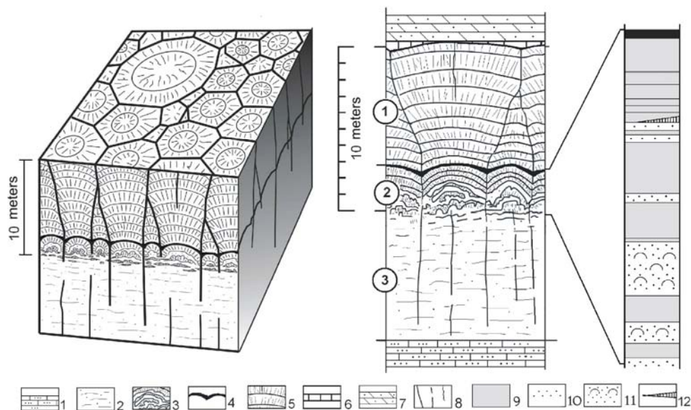
Рис. 1. Блок-диаграмма и разрез гипсовой толщи тирасской свиты (междуречье рек Серет и Ничлава, с. Алексинцы, пещера Мушкарова яма). Цифры в кружках – пакки гипсов. 1 – известняки биогермные багрянковые песчанистые с прослоями известковистых песчаников; 2 – гипсы скрыто-мелкозернистые, светло-серые с коричневатым оттенком; 3 – переслаивание скрыто-мелкозернистых светло-серых и крупно-гигантокристаллических коричневых гипсов; 4 – маркирующий прослой бентонитовых глин зеленовато-серых; 5 – гипсы крупно-гигантокристаллические коричневые; 6 – известняки пелитоморфные (ратинские); 7 – мергели зеленовато-серые с прослоями глин и песчаников; 8 – трещины в гипсовой толще; 9 – слои крупно и гигантокристаллических гипсов; 10 – слои скрыто-мелкозернистых гипсов; 11 – слои скрыто-мелкозернистых гипсов хлопьевидной «облачной» текстуры; 12 – маломощные линзы (до 5 см) бентонитовых глин оранжевого цвета.
